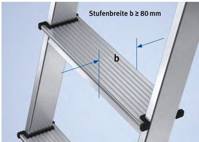
Abb. 8 Stufe
