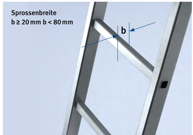
Abb. 9 Sprosse
