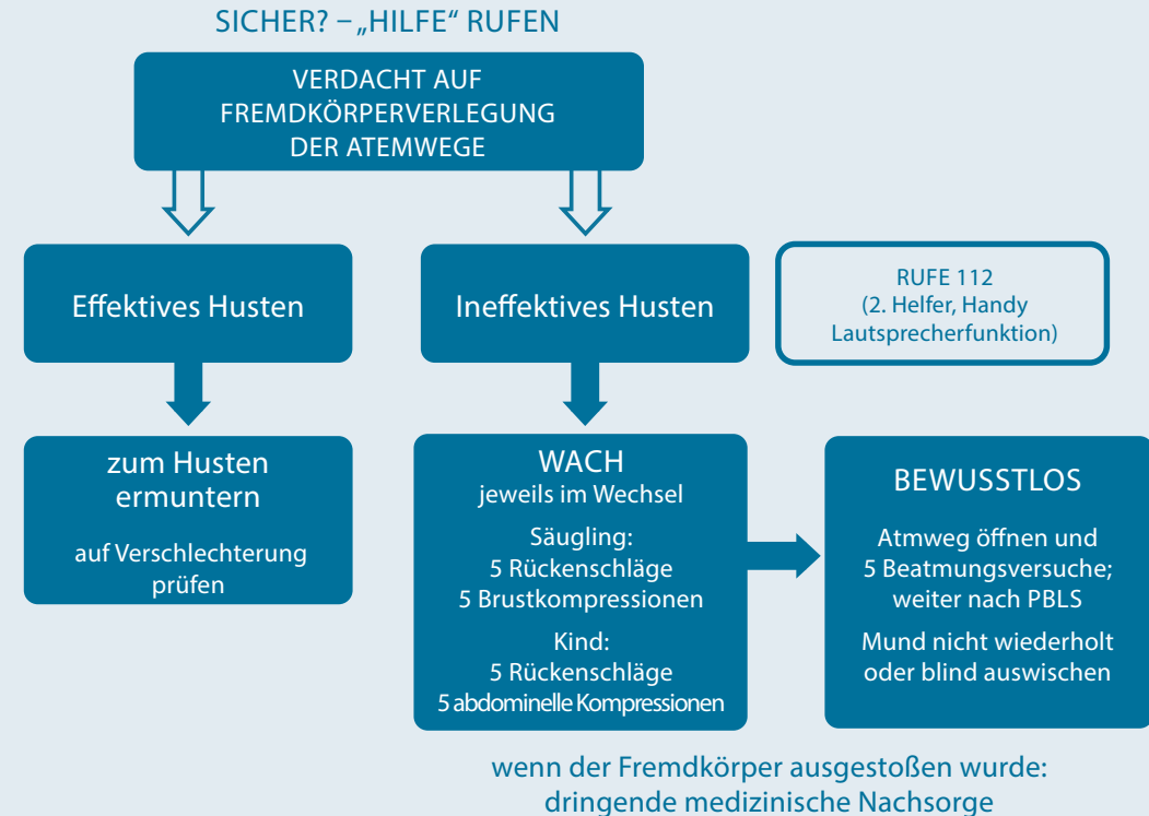
Abbildung 24 FBAO-Algorithmus
