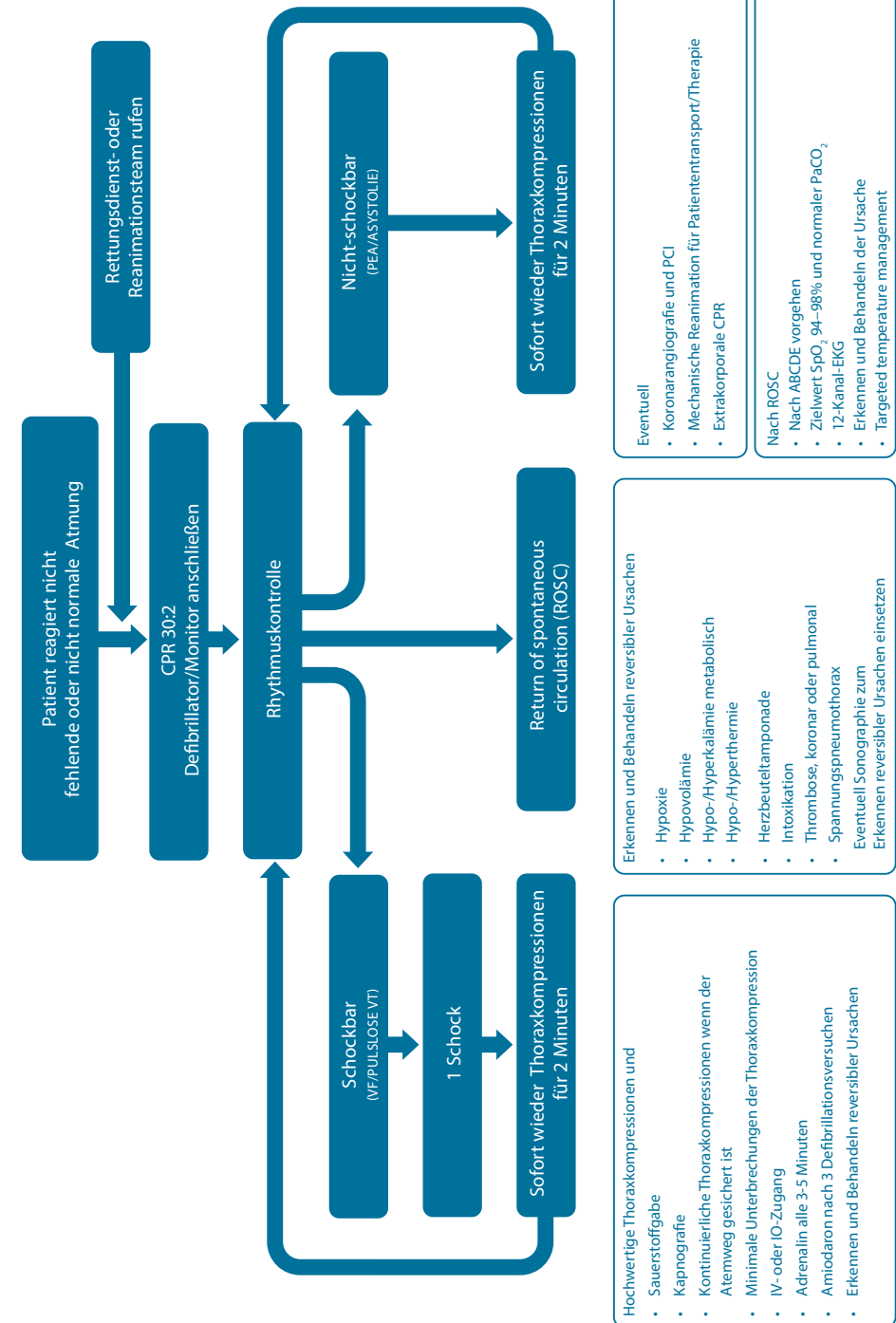
Abbildung 10 ALS-Algorithmus
